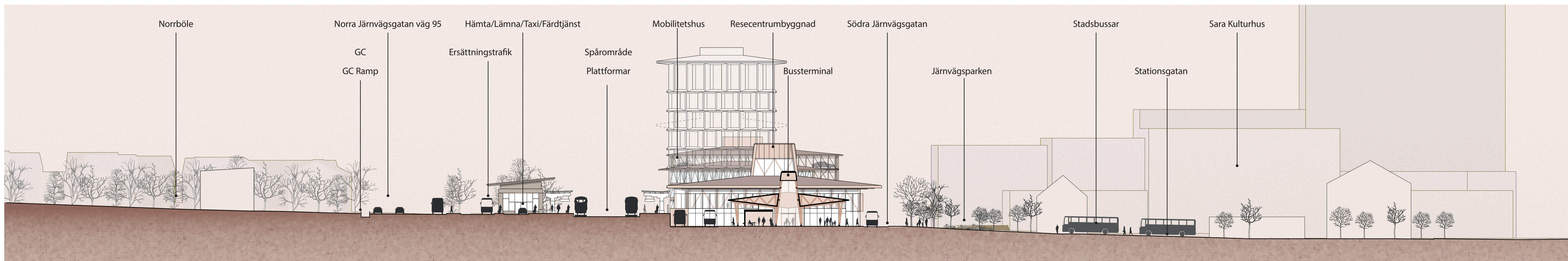
Elevation 3, 1:400 – Nord-sydlig riktning genom Bussterminalen vid Stationsgatan.
