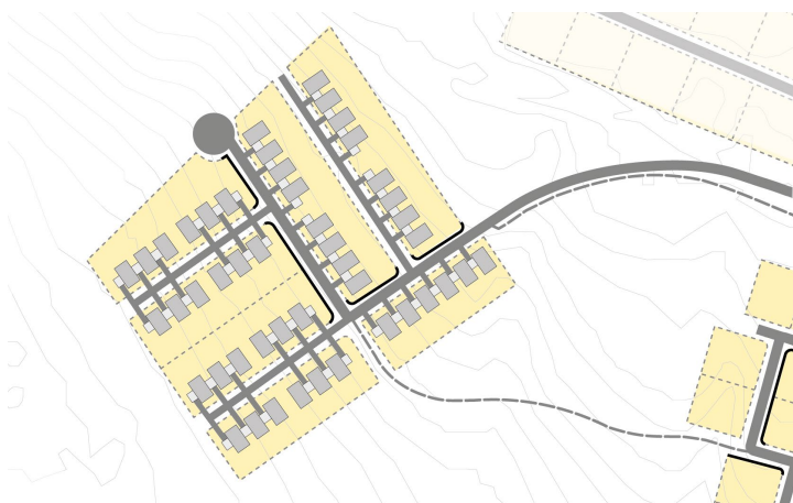
Figur 6. Illustrationen visar lämplig anslutning till kommande bostäder i radhusområdet i syfte att undvika schaktning i området.
