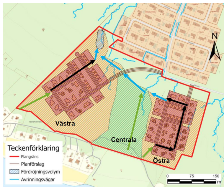
Figur 12. Karta över indelade delavrinningsområden och antagna rinnvägar inom dessa områden. Gröna pilar = avrinning på mark, svarta pilar = avrinning i ledningsburet system, blå pilar = avrinning i svackdike.
