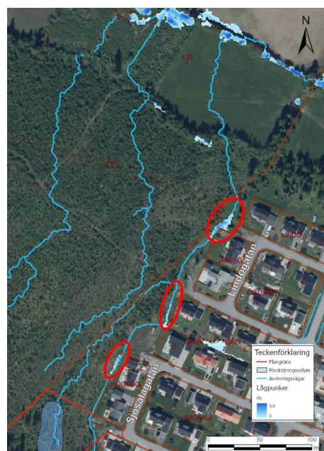
Figur 13. Befintlig avrinning nedströms planområdet. Röda ellipser visar lågpunkter där vatten riskerar att stiga till marknivå vid händelse av skyfall.
