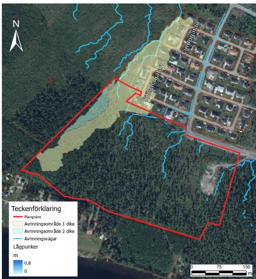
Figur 18. Befintliga avrinningsområden för diket nedströms planområdet.
