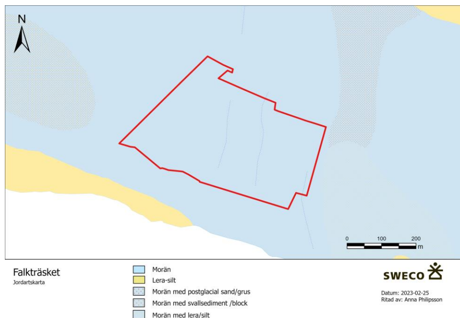
Figur 3. Jordartskarta. Information hämtad från SGU (2022).
