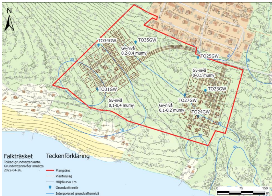
Figur 5. Interpolerade grundvattennivåer (blå linjer) i Falkträsket utifrån uppmätta värden 2022-04-26. Grå linjer är höjdkurvor från höjdmodell i Scalgo LIVE.
