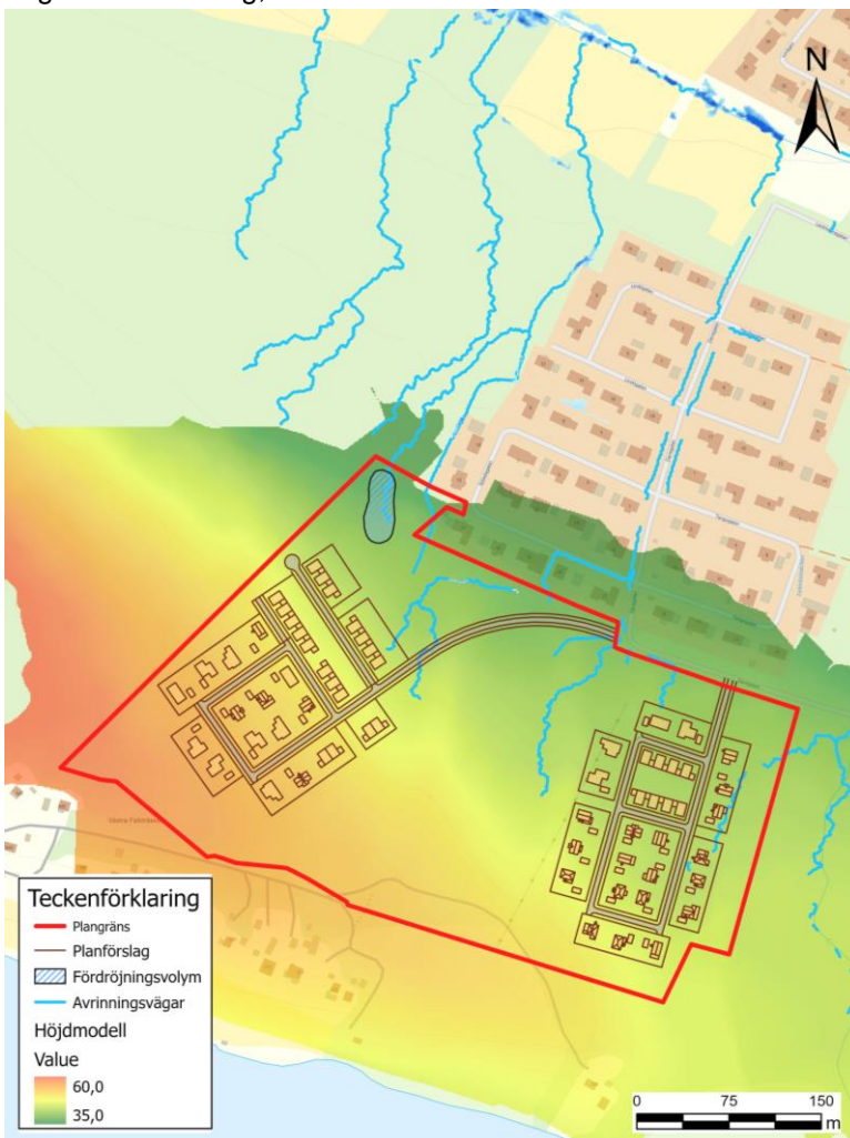
Figur 16. Detta område ligger i en lågpunkt nära detaljplanegränsen och bedöms även vara lämpligt utifrån tolkningar av grundvattennivåerna i området. Ytbehovet för den beräknade fördröjningsvolymen är ca 1250 m 2 , vilket motsvarar en reglerhöjd på 0,5 m. Därutöver tillkommer ytor för slänter och liknande.
