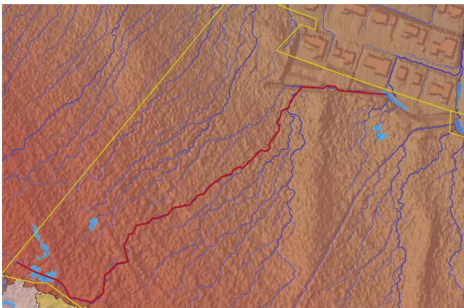
Figur 7. Längsta rinnsträckan för nuläget markerad med röd linje.
