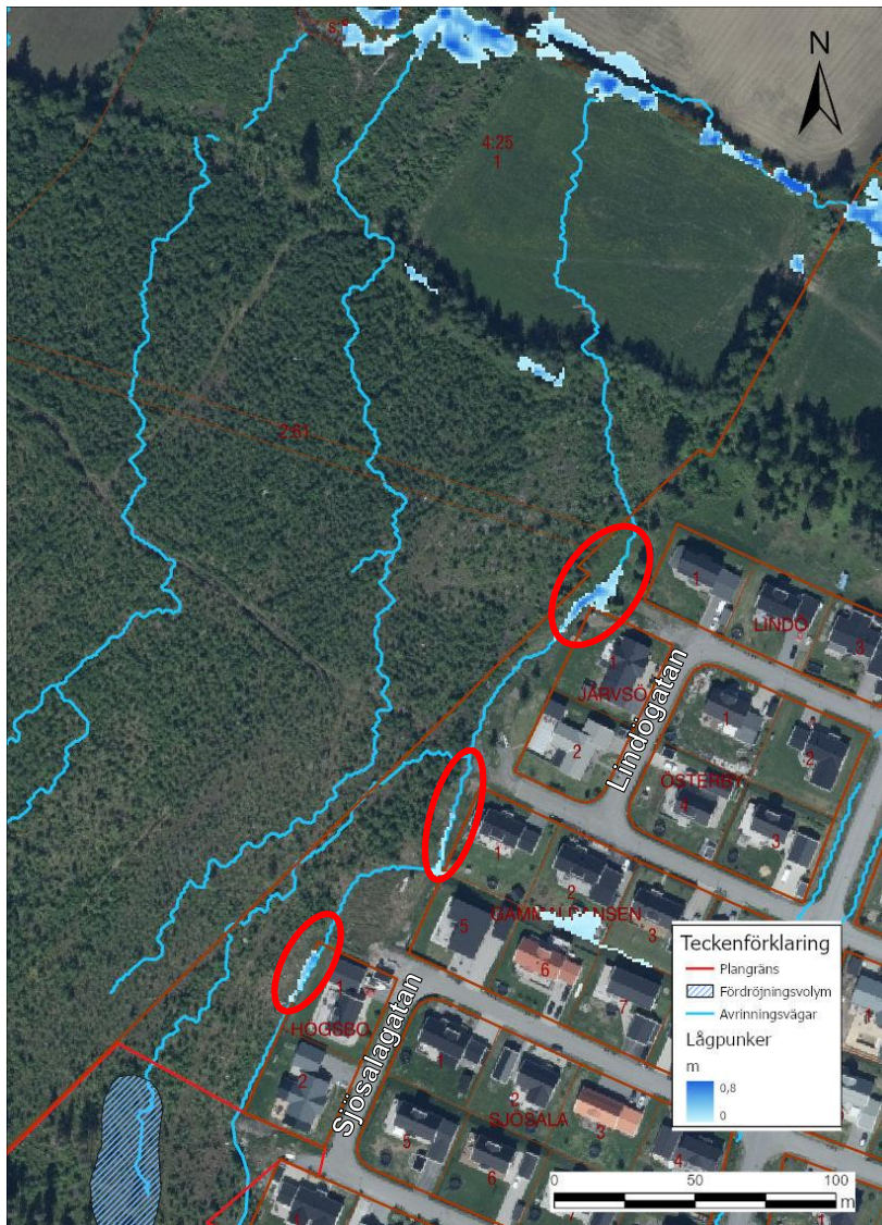
Figur 17. Befintlig avrinning nedströms planområdet. Röda ellipser visar lågpunkter där vatten riskerar att stiga till marknivå vid händelse av skyfall. Mörkröda linjer visar fastighetsgränser.
