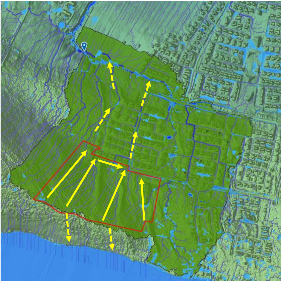
Figur 6. Avrinningsområdet som planområdet bidrar till. Gula pilar avser rinnriktning, plangränsen markerad i rött.
