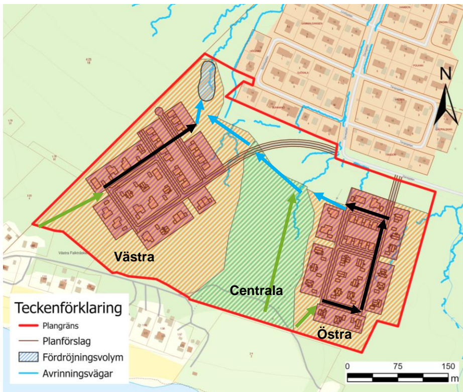
Figur 9. Karta över indelade delavrinningsområden och antagna rinnvägar inom dessa områden. Gröna pilar = avrinning på mark, svarta pilar = avrinning i ledningsburet system, blå pilar = avrinning i svackdike.
