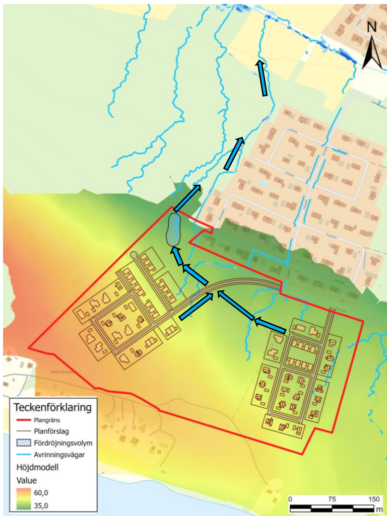
Figur 16. Skiss över planförslaget med höjddata i bakgrunden där grönt avser lägre markhöjder och rött avser högre markhöjder. Skrafferad markering avser lämpligt område för fördröjning. Blåa pilar avser schematiskt placerade rinnvägar för diken till och från fördröjningsanläggningen.
