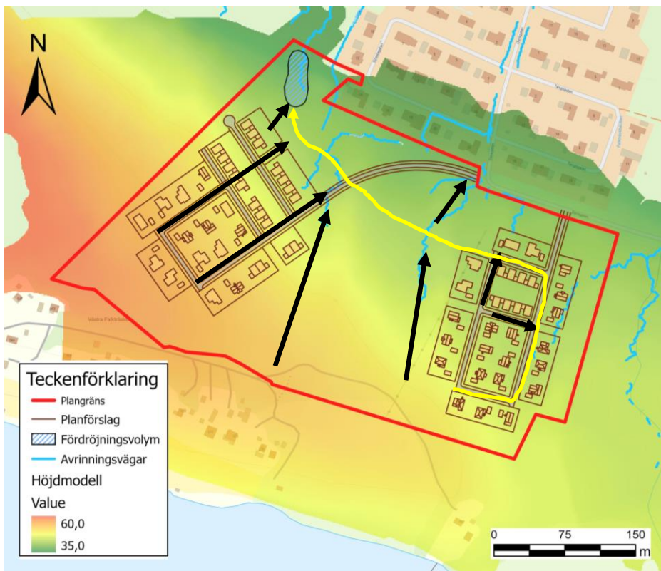
Figur 8. Förslag på utformning av planområdet. Gul linje visar längsta rinnväg genom planområdet. Svarta pilar visar generell avrinningsriktning.
