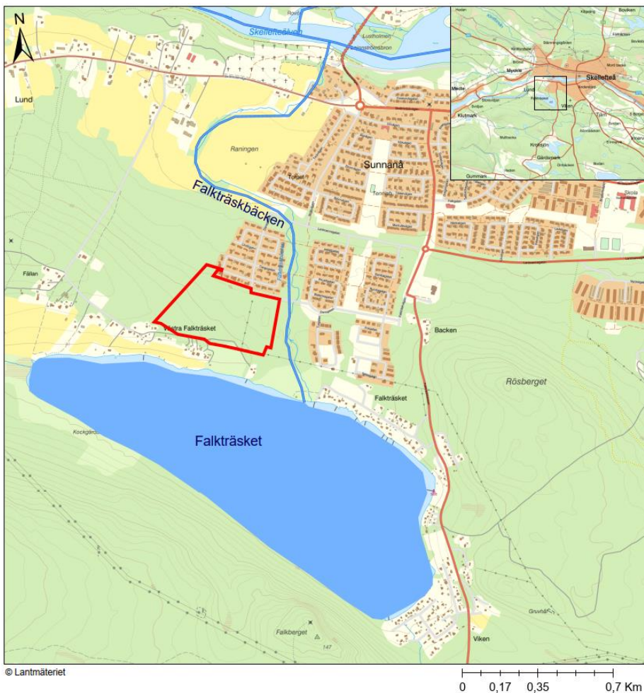
Figur 4. Figuren visar mottagande vattenförekomst Falkträskbäcken och dess läge i förhållande till planområdet (markerat med röd linje).
