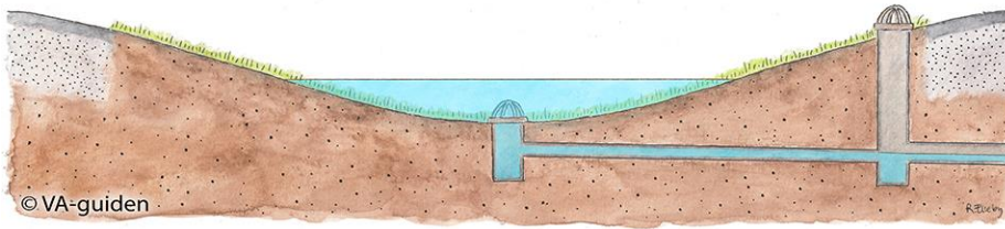
Figur 15. Principskiss för överdämningsyta / torr damm. Bild hämtad från www.vaguiden.se.
